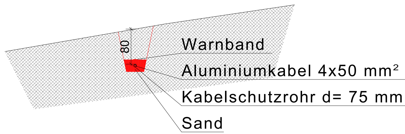
Regelquerschnitt M= 1:50
