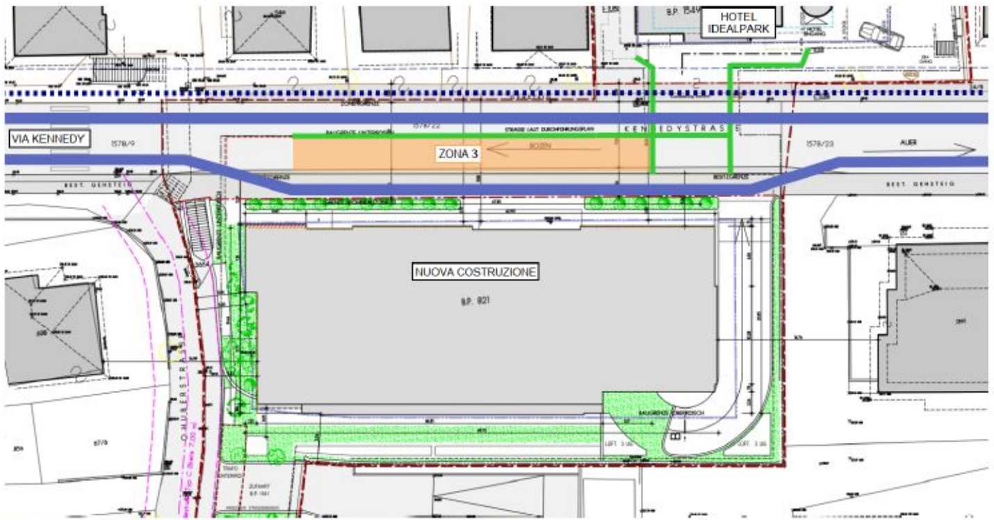
Deviazione corsie nella Fase 3 durante lo scavo e la realizzazione del solaio.
