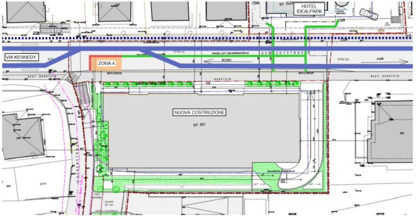
Deviazione corsie nella Fase 4.
