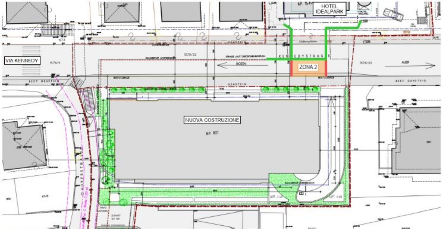
Realizzazione pali, scavo e solai nella Zona 2.
